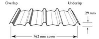
Trimdek®
